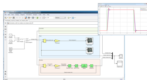
Simulation « Hardware in the loop » période d'échantillonnage jusqu'à 50 \mu s
