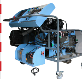
banc moteur
